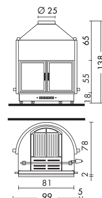
IDRO 70 - 100 - standardowe drzwiczki dwuskrzydłowe
