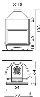
IDRO 50 - jednoskrzydłowe drzwiczki otwierane do wewnątrz
