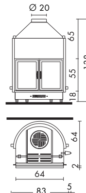
IDRO 70 - 100 - standardowe drzwiczki dwuskrzydłowe
